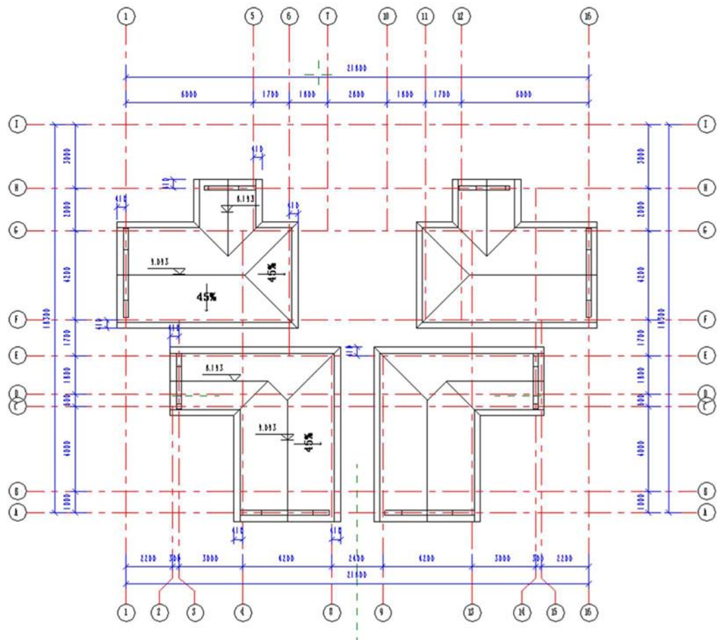
屋顶层平面图
