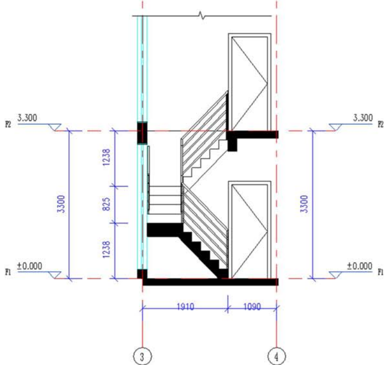
楼梯剖面
