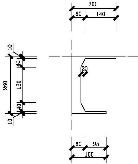
东立面轮廓 1:20
